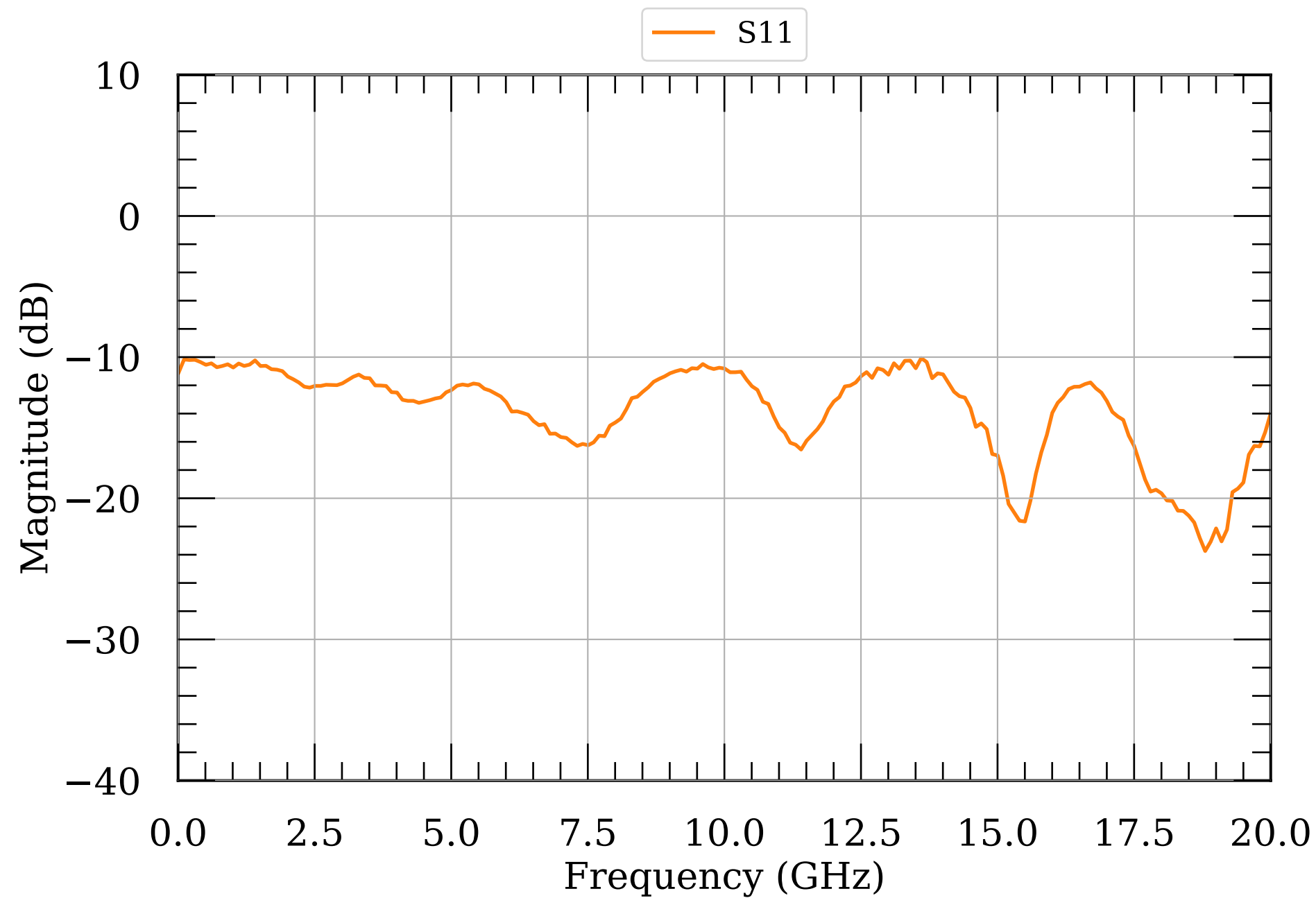
LNA S-params module095
